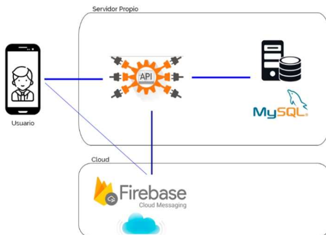
Figura 5. Arquitectura cliente servidor
