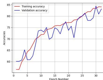
Fig. 5. Validación de Accuracy según modelo VGG-16
